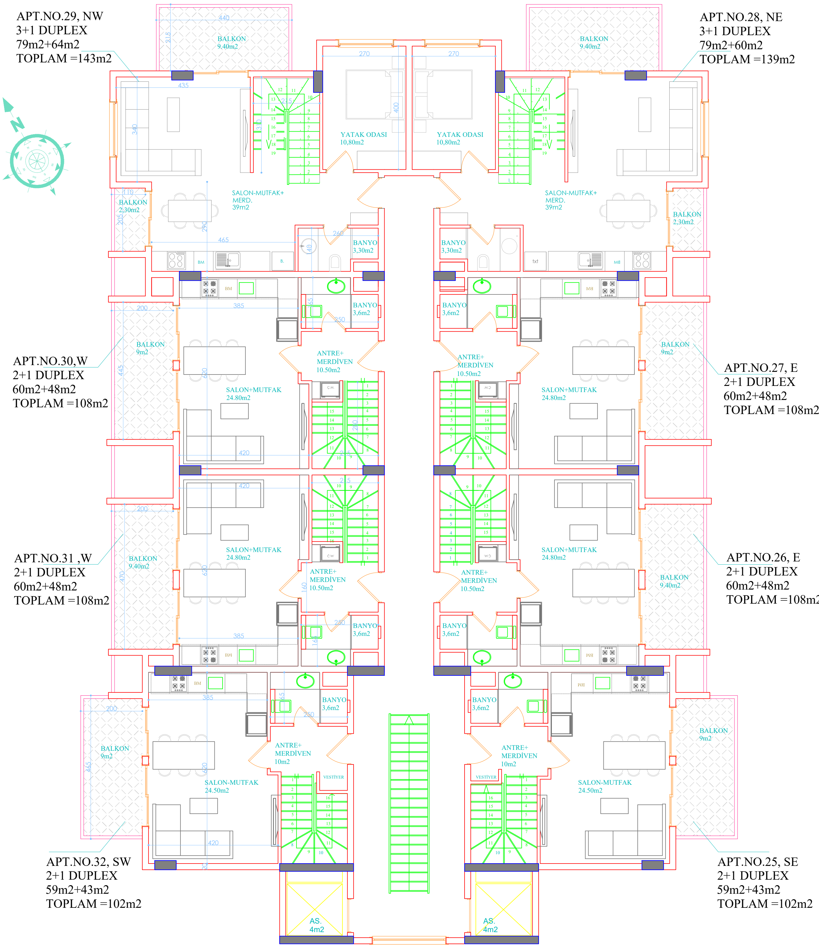
3. KAT PLANI
