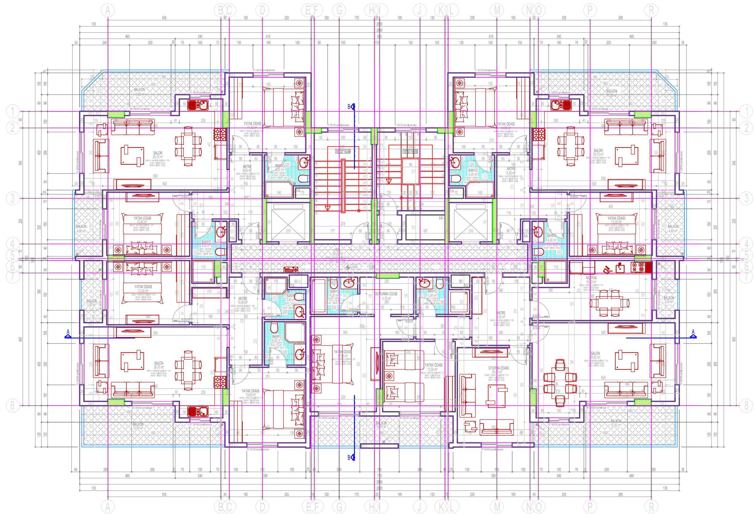
4. KAT PLANI ÖLÇEK: 1/50
